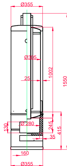
KUPAONSKA PEĆ "IVA" 70 LITARA
