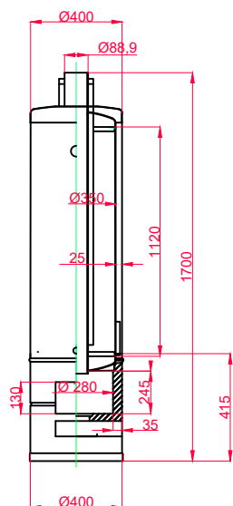
KUPAONSKA PEĆ "IVA" 100 LITARA
