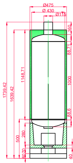
KUPAONSKA PEĆ "IVA" 150 LITARA
